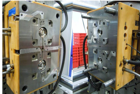
Düsenseite
